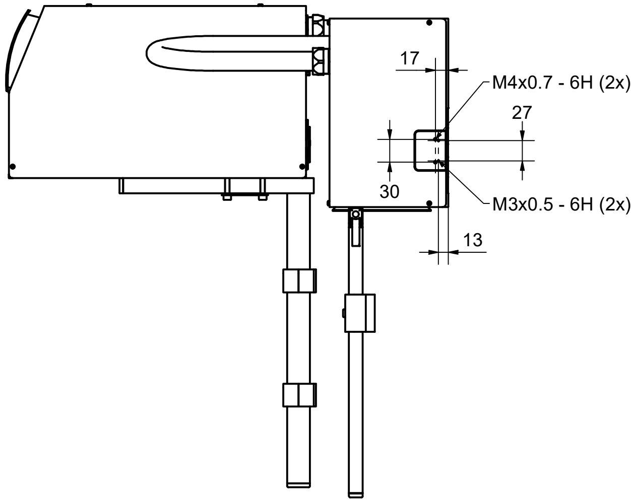
Seitenansicht von links side view left
