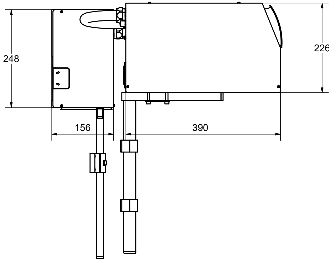
Seitenansicht von rechts side view right
